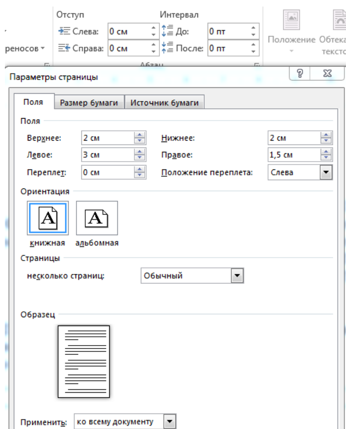
Рисунок 3.1 – Параметры страницы
